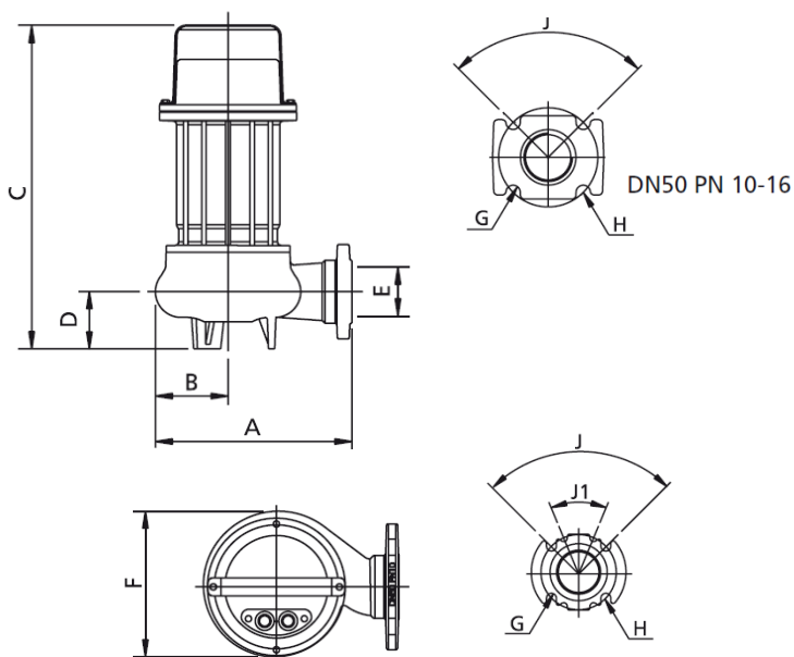
Bild 2 (Druckanschluss horizontal)
